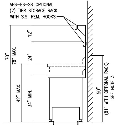
END ELEVATION
